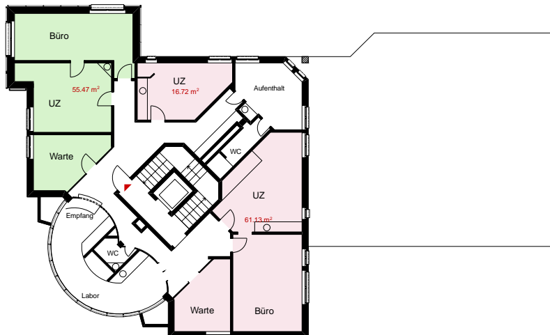
Gladbachstrasse 95 - EGID 2373708 1. Obergeschoss
